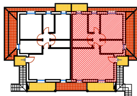
INQUADRAMENTO GENERALE Piano Primo
