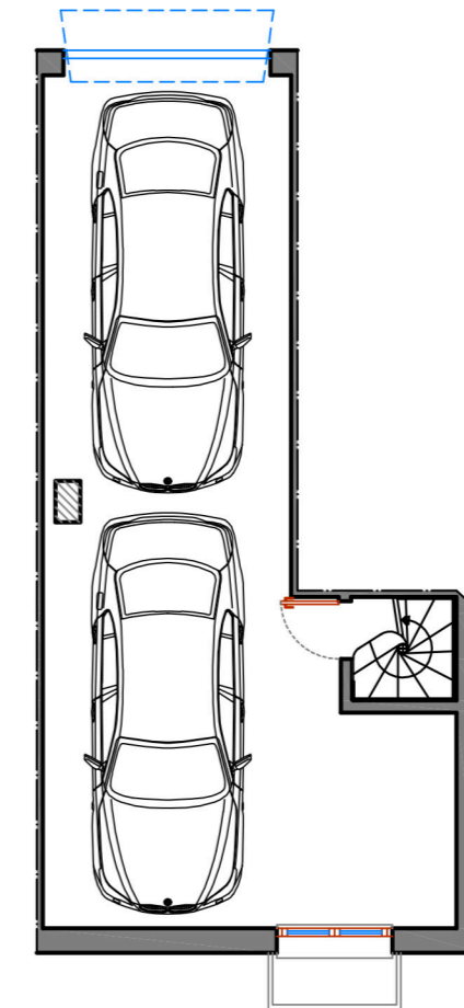
PIANO INTERRATO Scala 1:100
