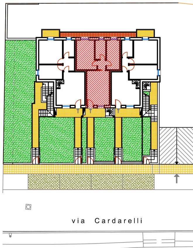
INQUADRAMENTO GENERALE Piano Terra
