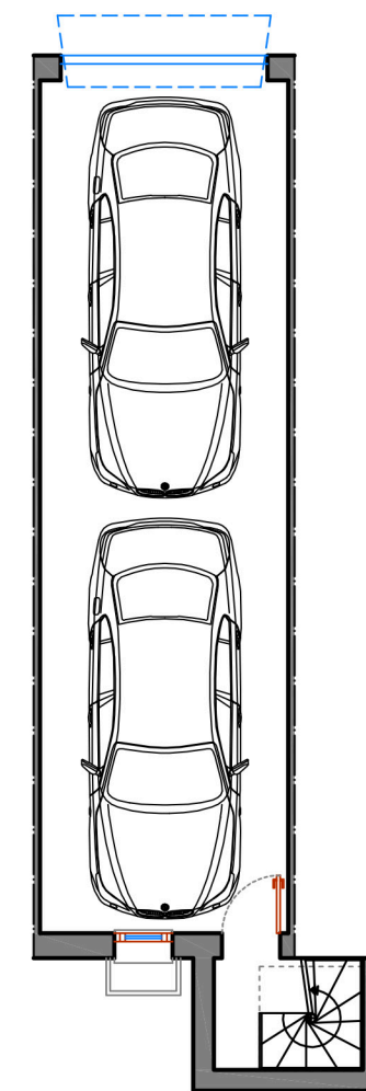
PIANO INTERRATO Scala 1:100
