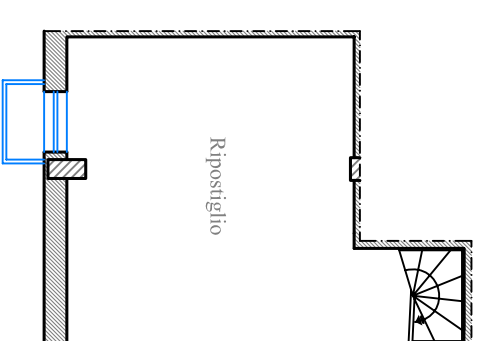
PIANO INTERRATO Scala 1:100
